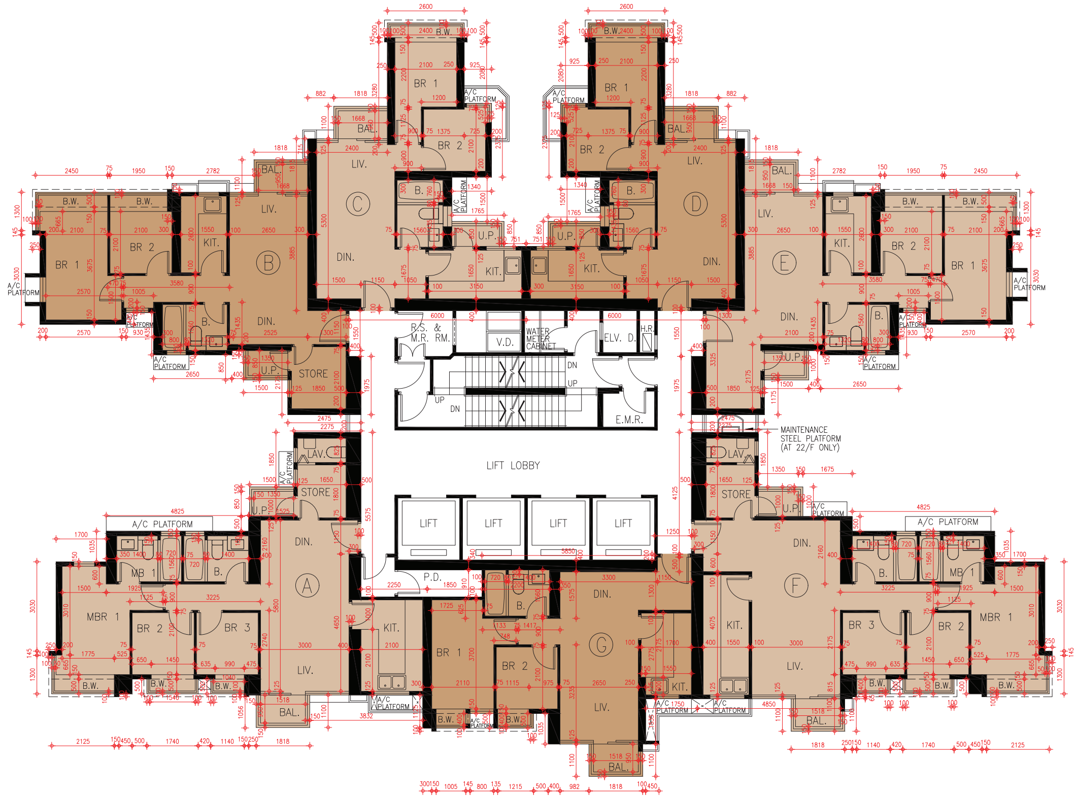
Tower 9 7/F - 13/F & 15/F - 22/F Floor Plan 第9座7樓至13樓及15樓至22樓樓面平面圖
