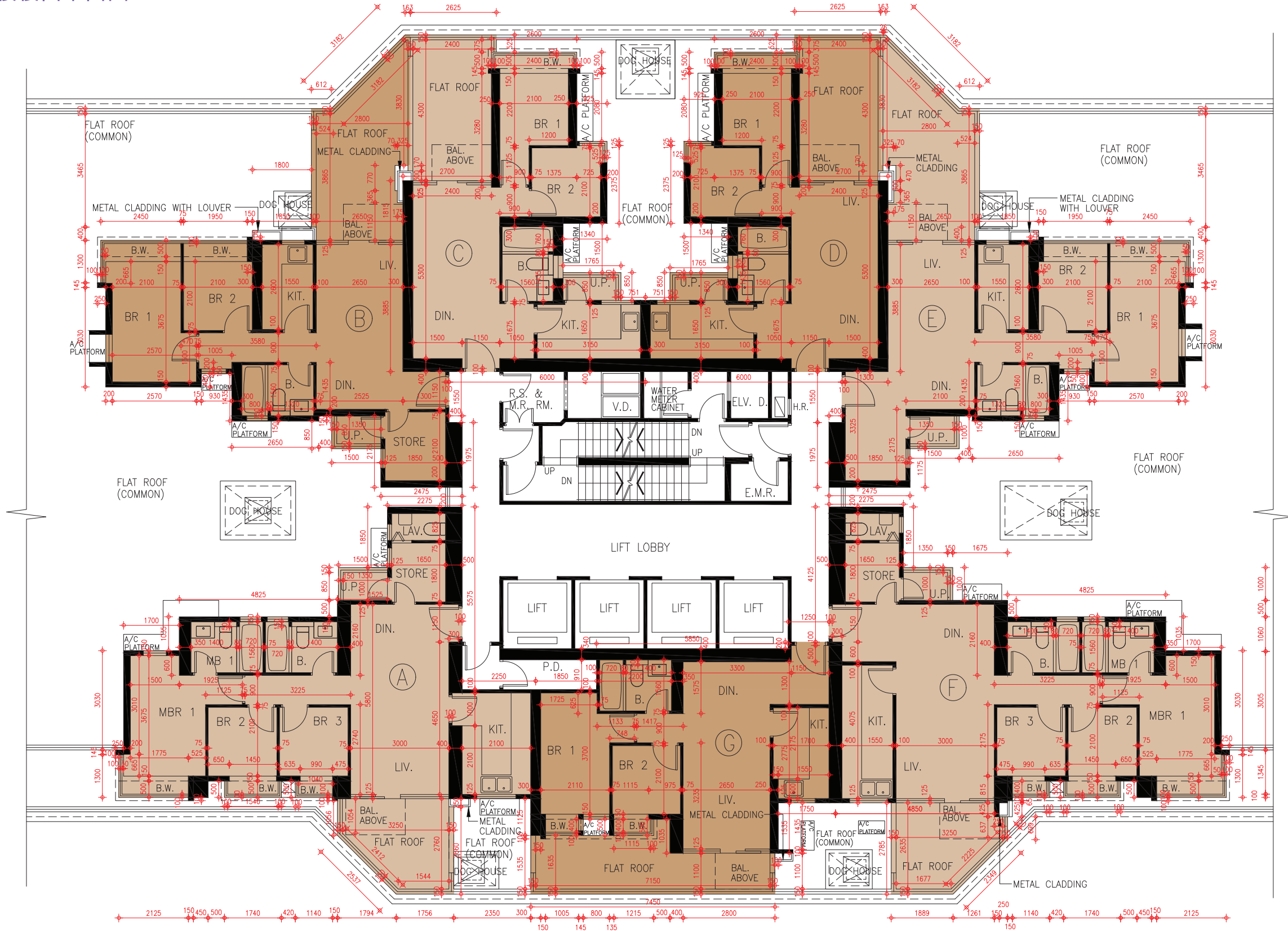
Tower 9 6/F Floor Plan 第9座6樓樓面平面圖
