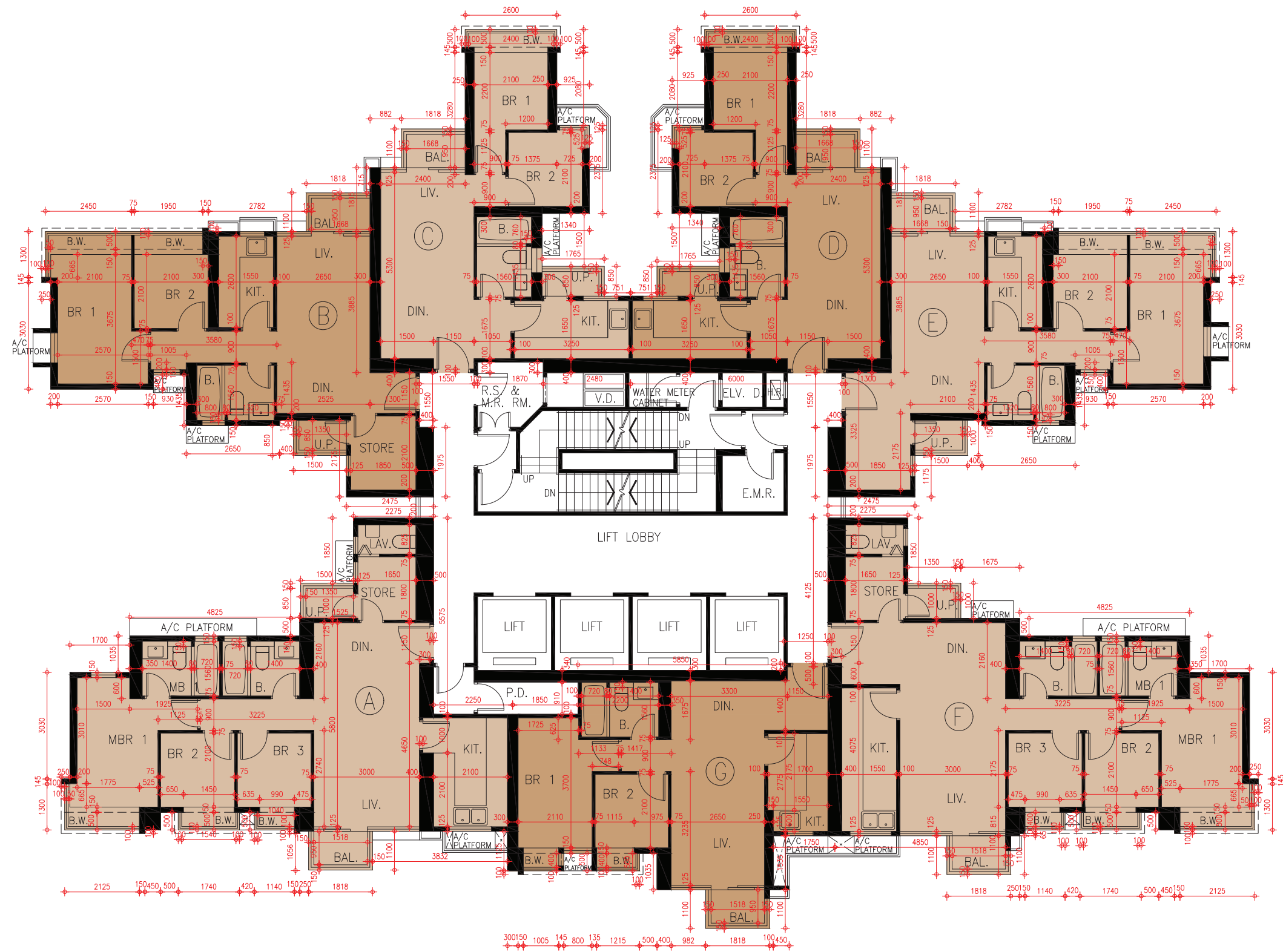
Tower 9 45/F - 48/F Floor Plan 第9座45樓至48樓樓面平面圖
