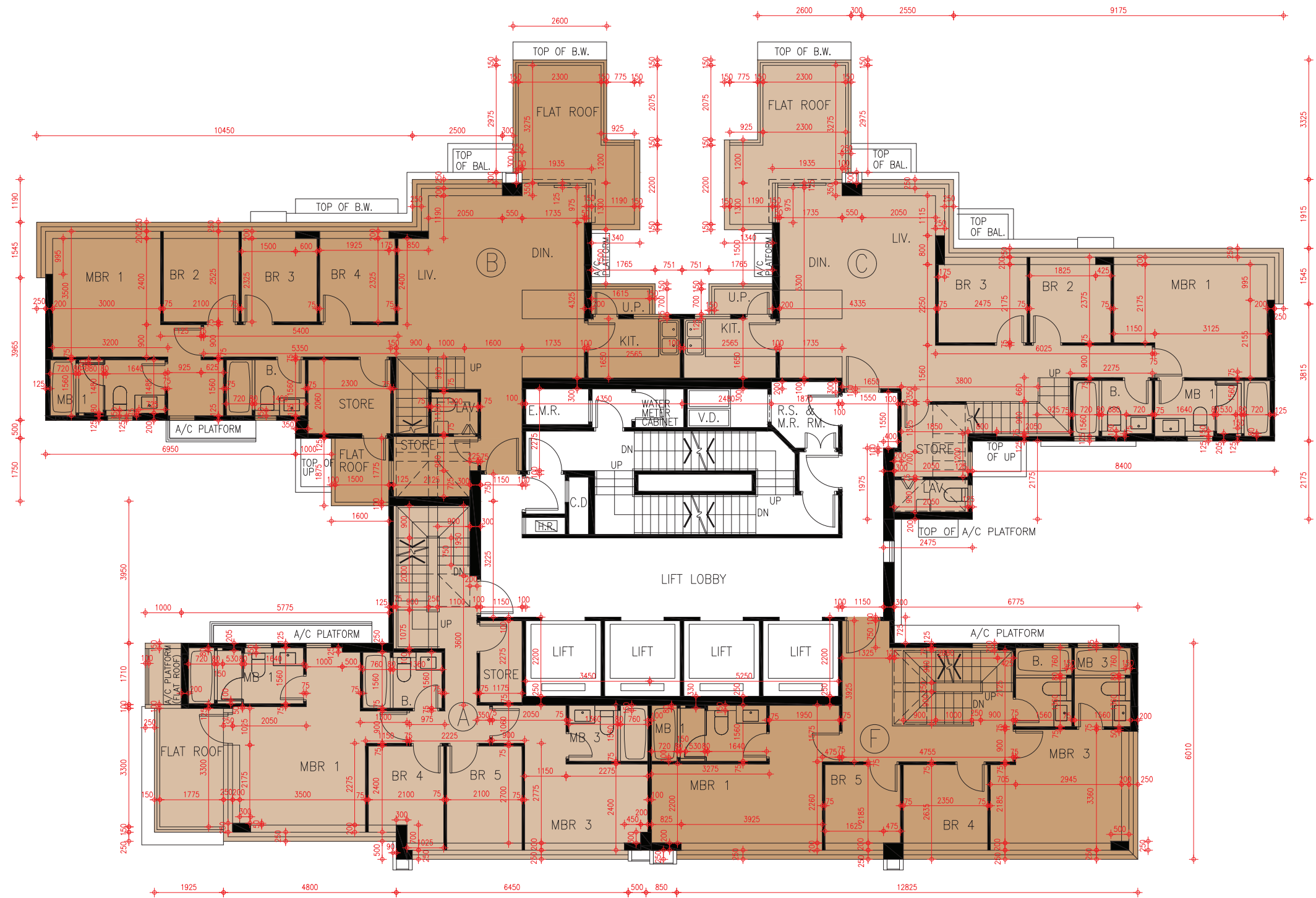
Tower 10 51/F Floor Plan 第10座51樓樓面平面圖
