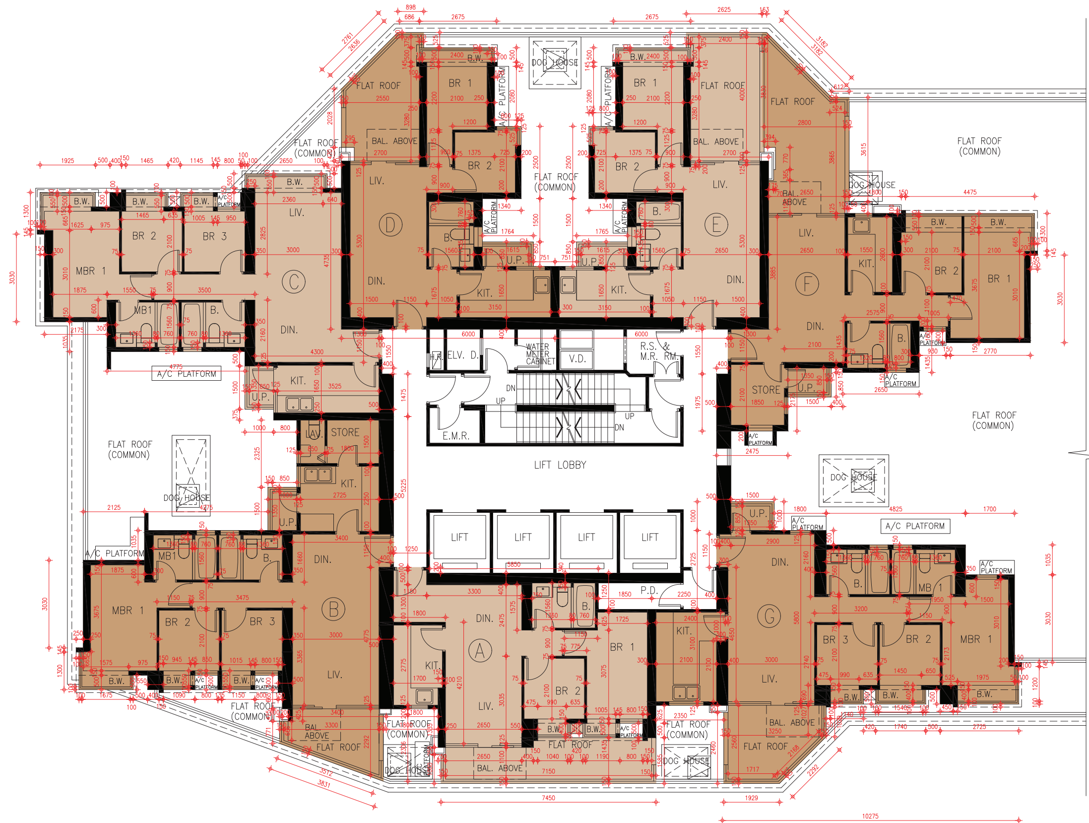
Tower 10 6/F Floor Plan 第10座6樓樓面平面圖
