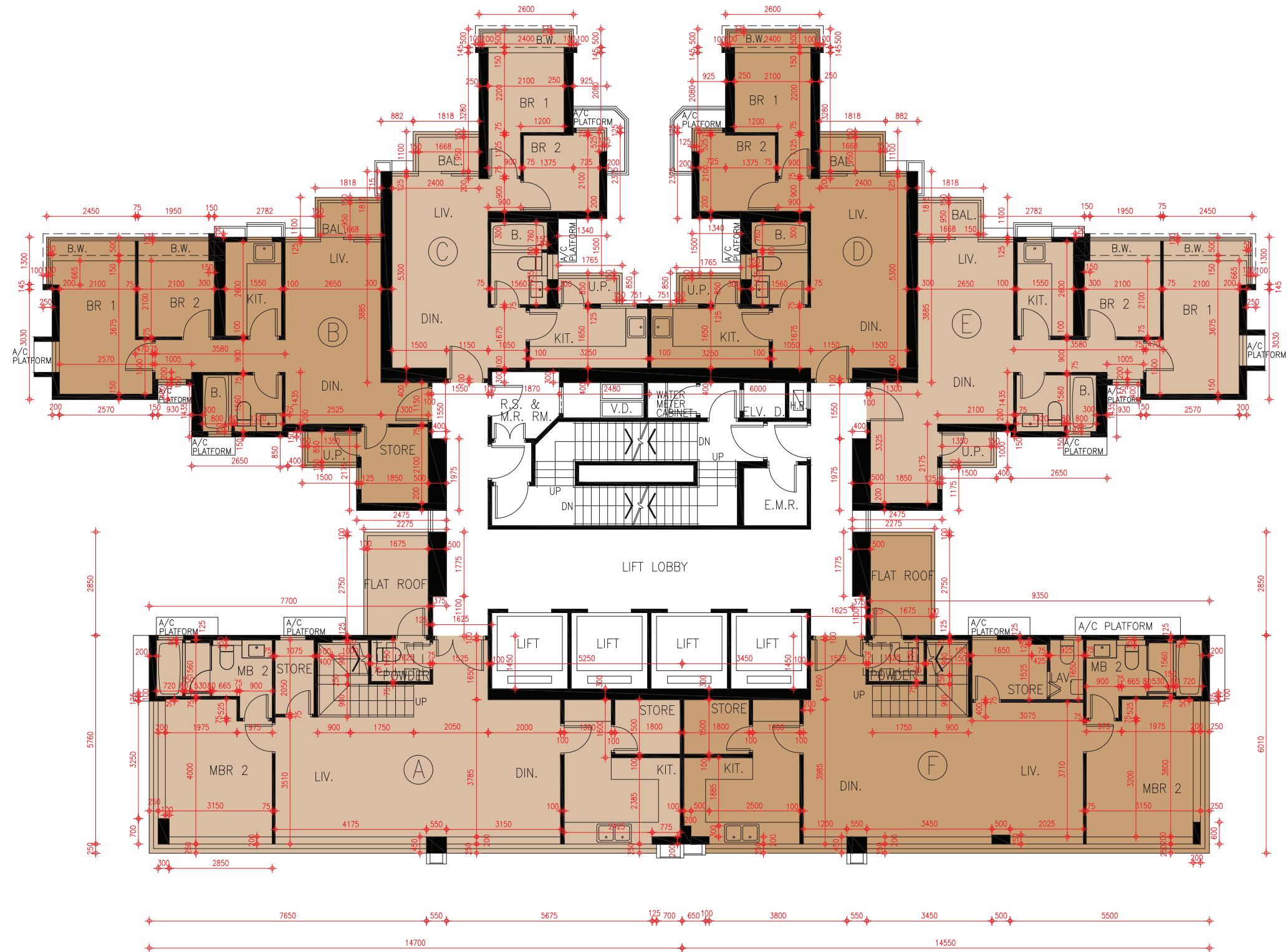
Tower 9 50/F Floor Plan 第9座50樓樓面平面圖
